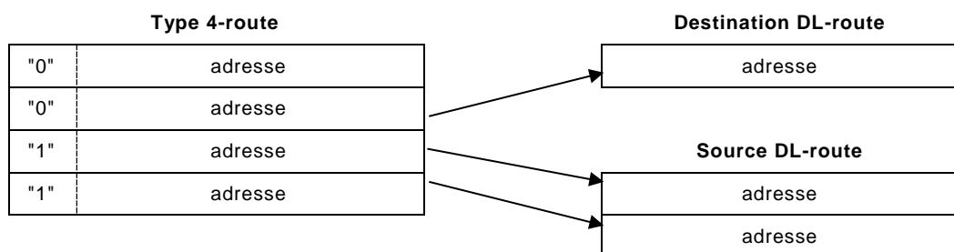
Figure 20 – Génération d'une DL-route Extended
