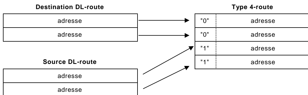
Figure 17 – Génération d'une Type 4-route Extended
