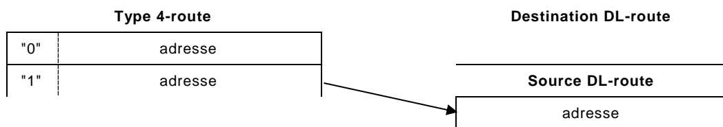
Figure 19 – Génération d'une DL-route Simple
