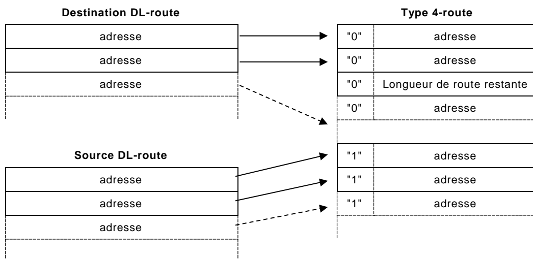
Figure 18 – Génération d'une Type 4-route Complex et IP
