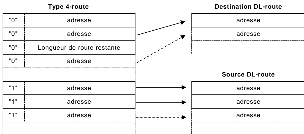
Figure 21 – Génération d'une DL-route Complex et IP
