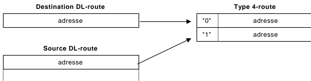
Figure 16 – Génération d'une Type 4-route Simple
