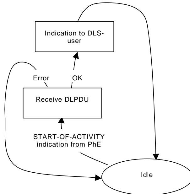
Figure 4 – Diagramme d'états de DLE pour des DLPDU acquittées non confirmées
