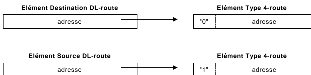
Figure 15 – Indicateur de source/destination
